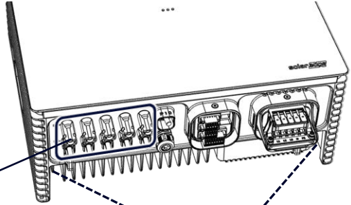
M5 x 16 T15-Schraube 2,7 Nm Erdung (PE)
